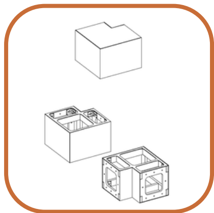
2-way hoeelement
